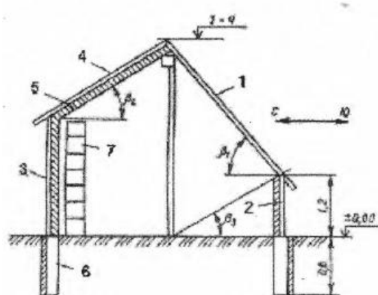
Рис. 2. Отдельно стоящая солнечная теплица:
